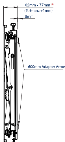
SEITENANSICHT GESCHLOSSEN
