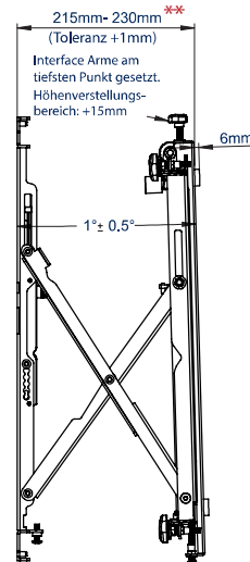
SEITENANSICHT VERLÄNGERT
