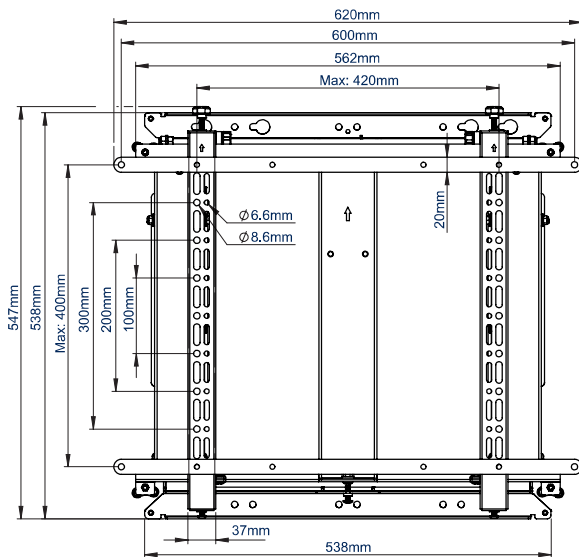
VORDERANSICHT MIT ADAPTER ARMEN
