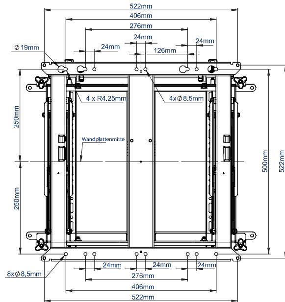
RÜCKANSICHT
